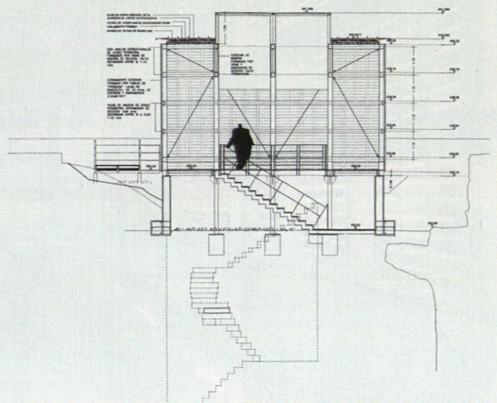
05 - SECCION CONSTRUCTIVA DE ENTRADA AL PABELLÓN
