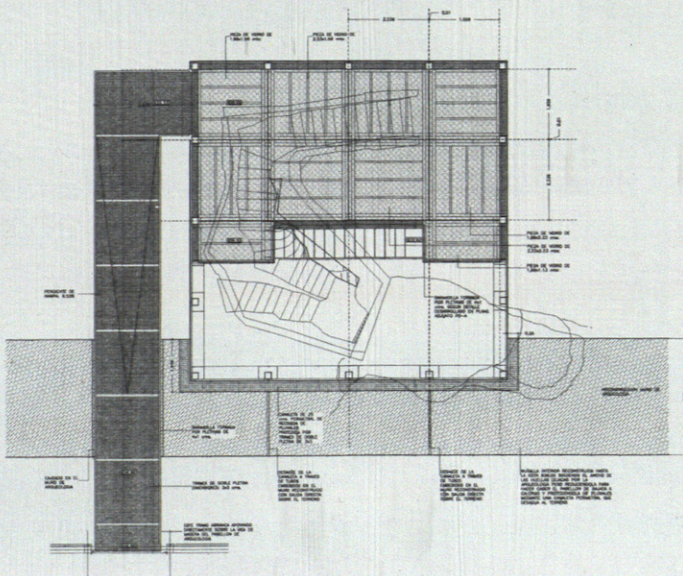
04 - PLANTA DEL PABELLÓN
